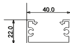
■ LISSE BARREAUDAGE GC4026
