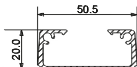
■ LISSE TÊTE DE POTEAU GC4021N
