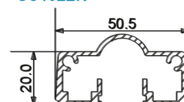
● LISSE TÊTE DE POTEAU GC4022N
