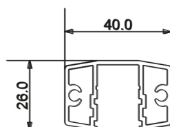
■ LISSE VITRAGE GC4028A
